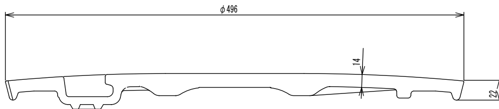
A-A' 断面図
