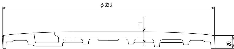
A-A' 断面図
